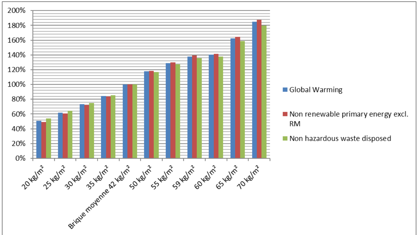
Graphique illustrant la variabilité des résultats d'impacts environnementaux sur 3 indicateurs en fonction de la variation de la masse de briques de cloison au mètre carré
